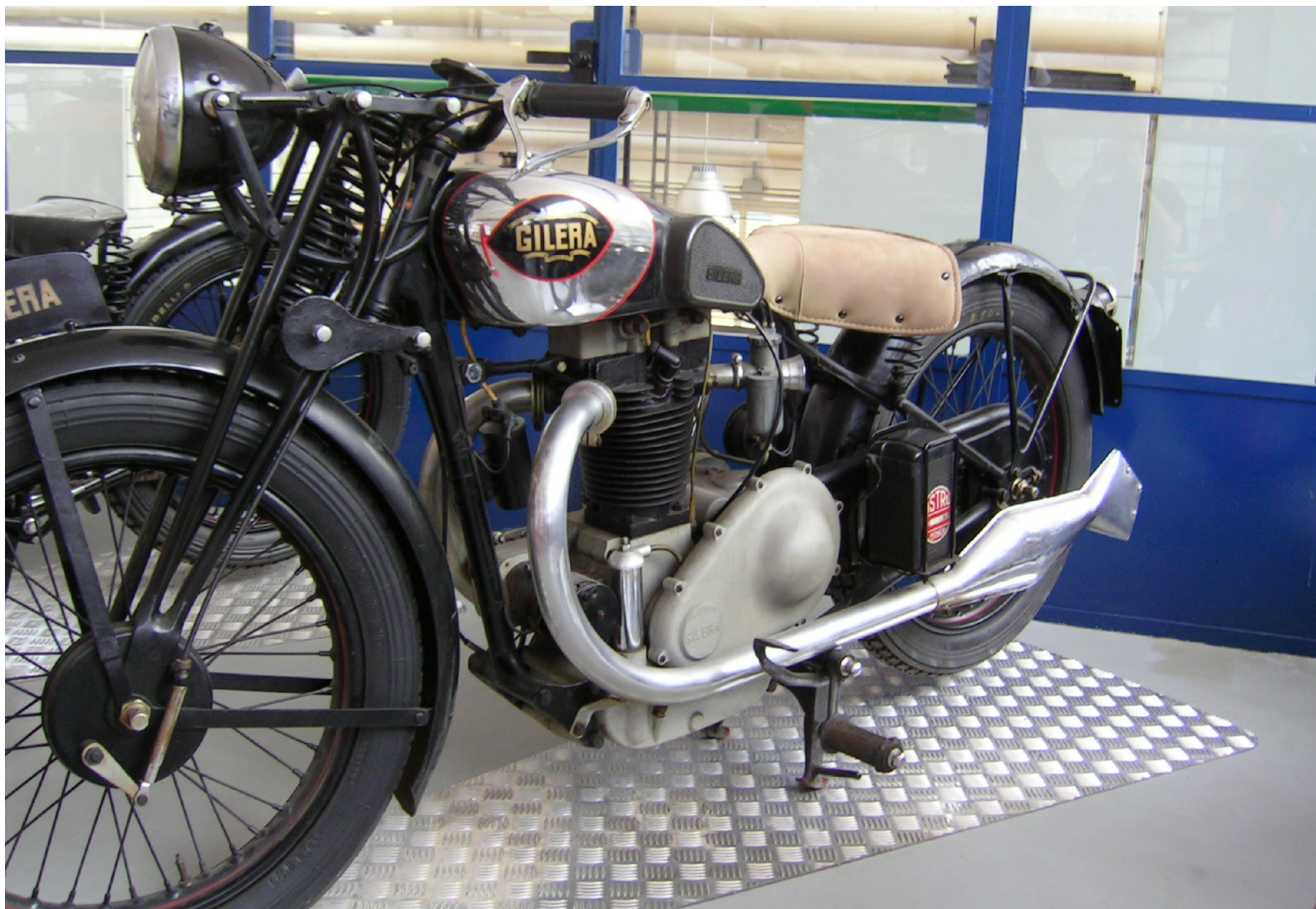
GILERA VT 500 1934 (quattro bulloni) 3 soupapes, 4 vitesses et graissage sous pression
