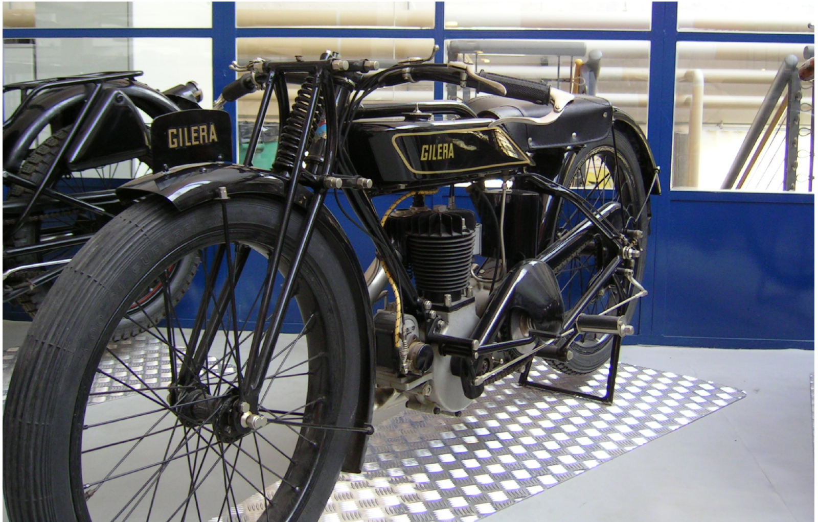
GILERA 500 Supersport 1928: Distribution enclose et graissage sous pression. Freins couplés avant/arrière sur la version tourisme.
